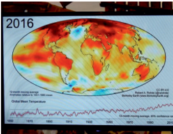
langfristige Temperatur-Veränderungen
